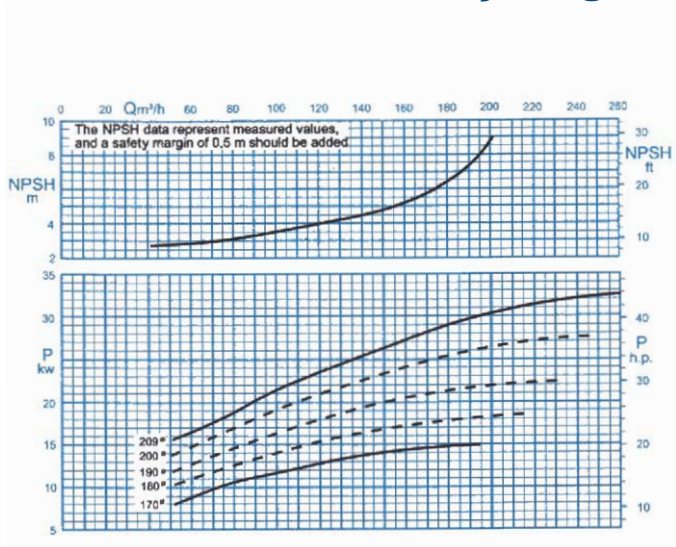
منحنی عملکرد
