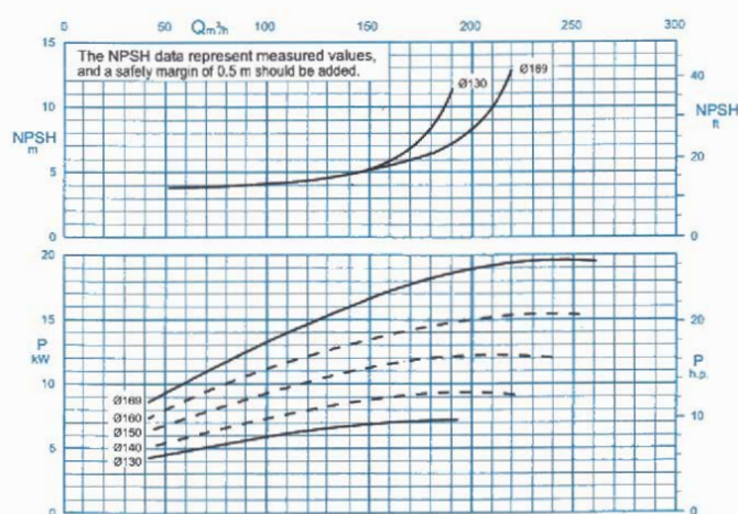
منحنی عملکرد
