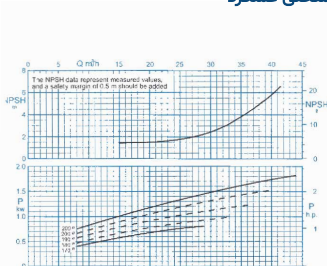
منحنی عملکرد
