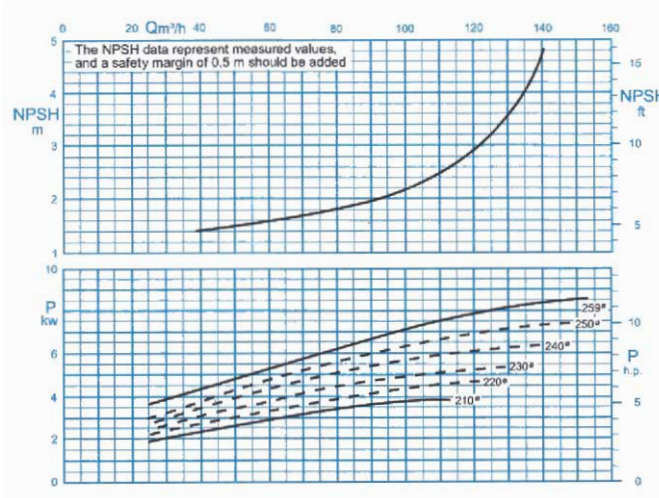
منحنی عملکرد
