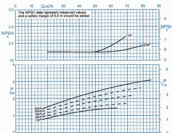
منحنی عملکرد
