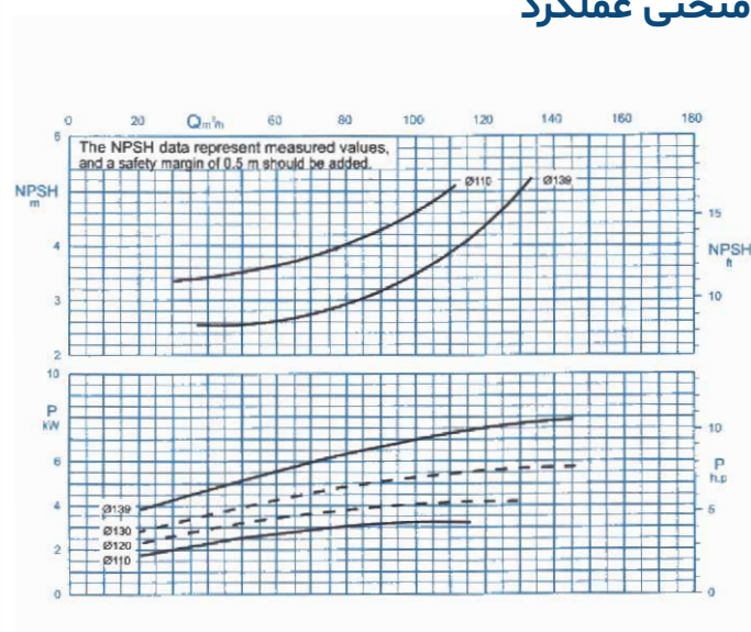
منحنی عملکرد
