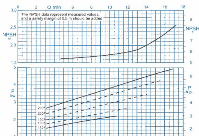
منحنی عملکرد
